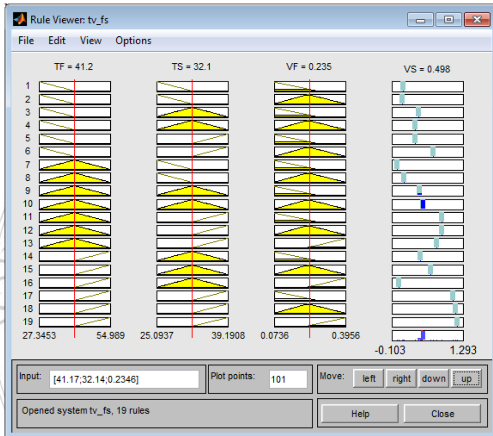
Fig. 11. Predicting values for BV.
